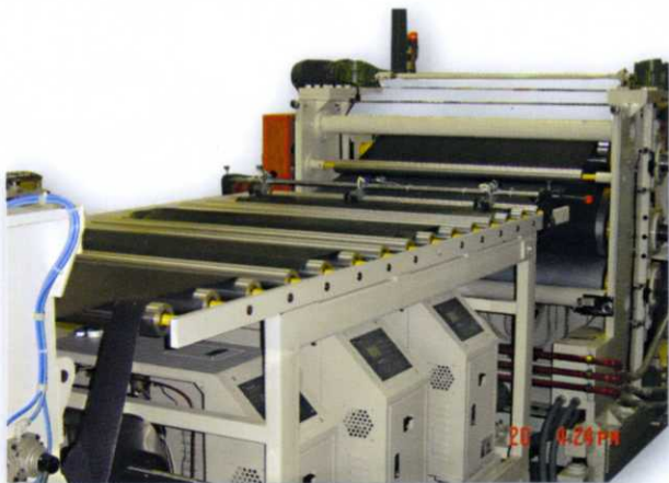
Roller Passage
