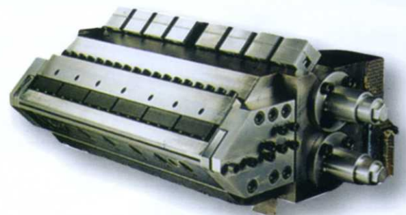
T-Die
